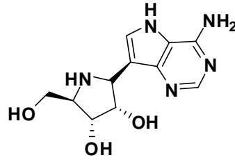
Galidesivir
