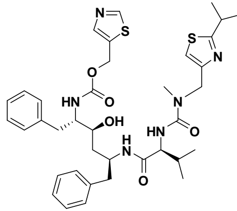
Ritonavir
